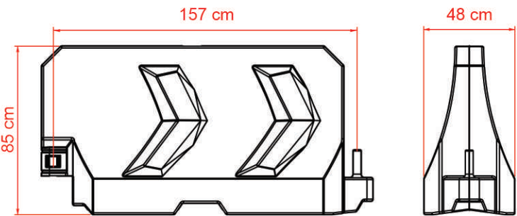
VISTA LATERAL
