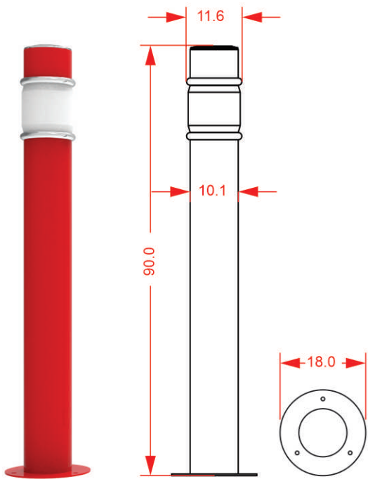
BOLARDO FIJO
