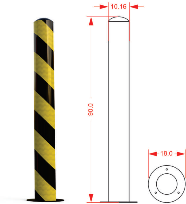
BOLARDO FIJO
