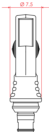
VISTA LATERAL
